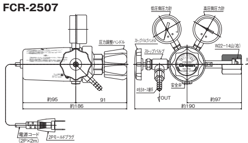
FCR-2507
