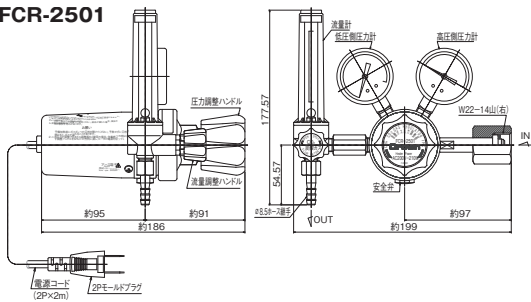
FCR-2501
